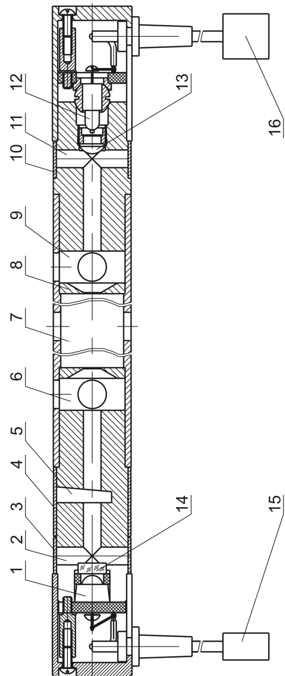
1- Фотодатчик (фотодиод); 2-Отверстие для очистки светофильтра; 3, 4-Шторка; 5-Гнездо для установки контрольного светофильтра; 6,9-Буферная камера; 7-Измерительная камера; 8-Диафрагма; 10-Шторка; 11-Отверстие для очистки оптической линзы; 12-Лампа; 13-Оптическая линза; 14-Светофильтр; 15, 16-Разъемы для подключения к плате обработки модуля контроля дымности
