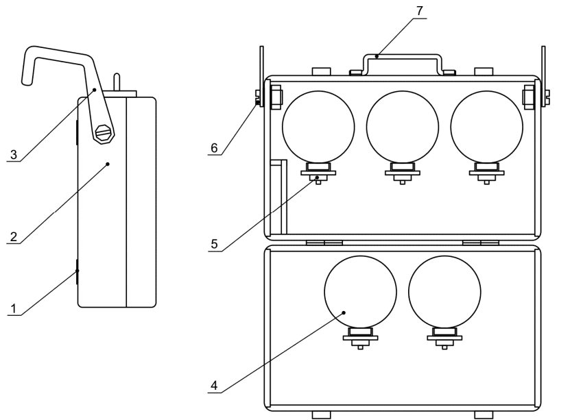
1-Накладка, 2-Ящик, 3-Скоба, 4-Манометр, 5-Штуцер манометра, 6-Винт, 7-Ручка
