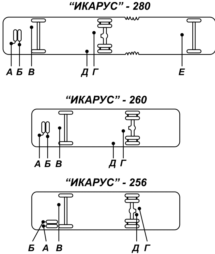
Рисунок 9 – Расположение контрольных клапанов на автобусах «Икарус»-280, «Икарус»-260, «Икарус»-256
